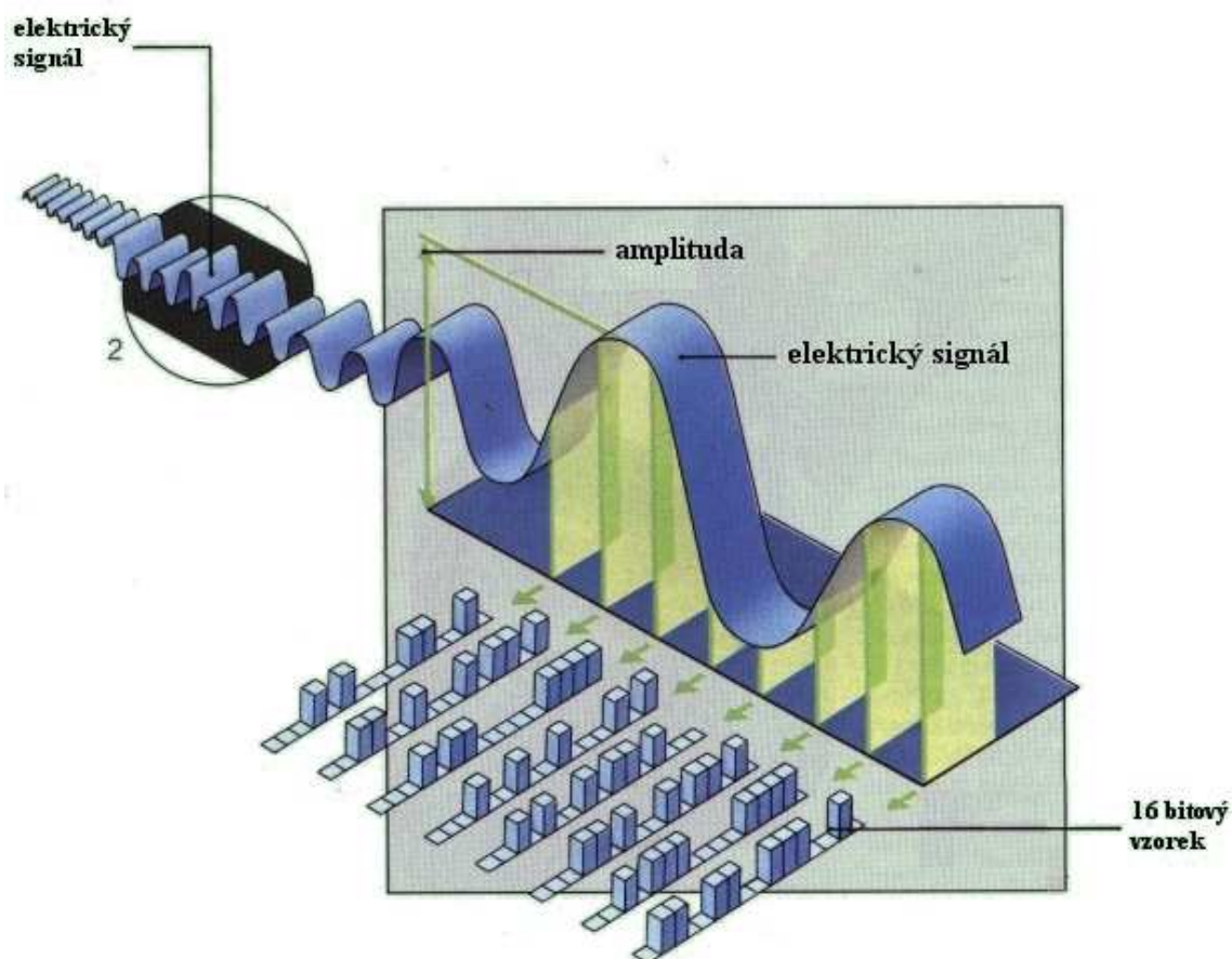
Obrázek 6.1: Digitalizace zvuku 2
