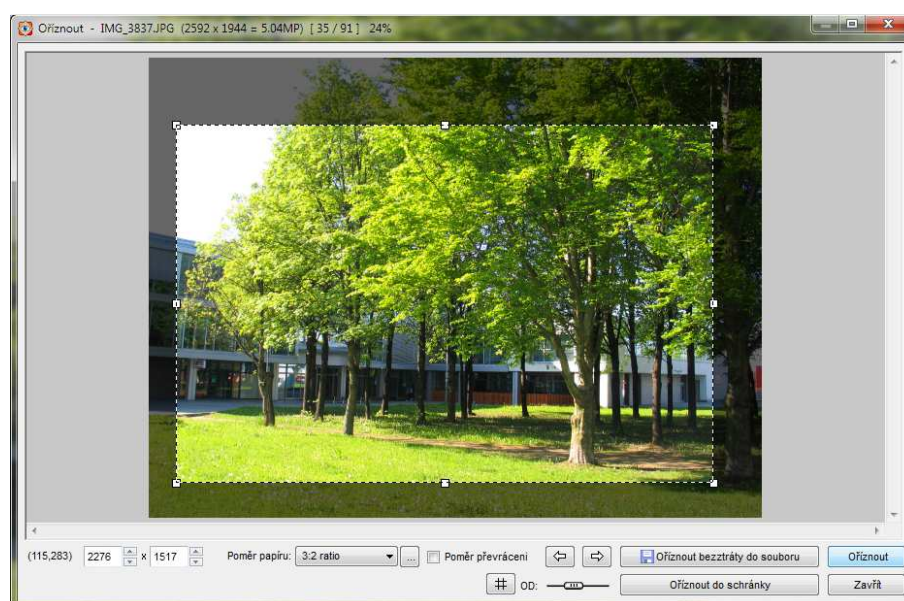
Obrázek 3.4: Oříznutí fotografie
