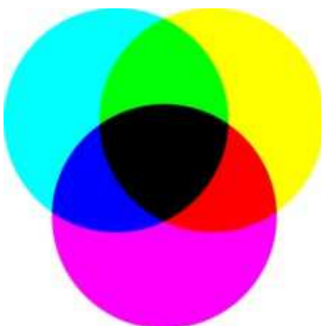
Obrázek 1.2: Model CMY
