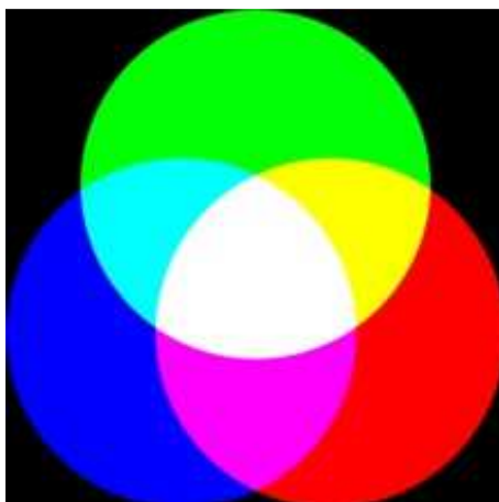
Obrázek 1.1: Model RGB
