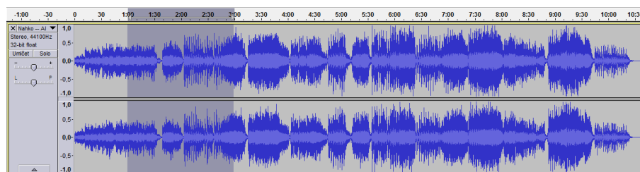
Obrázek 7.8: Vytvořený výběr
