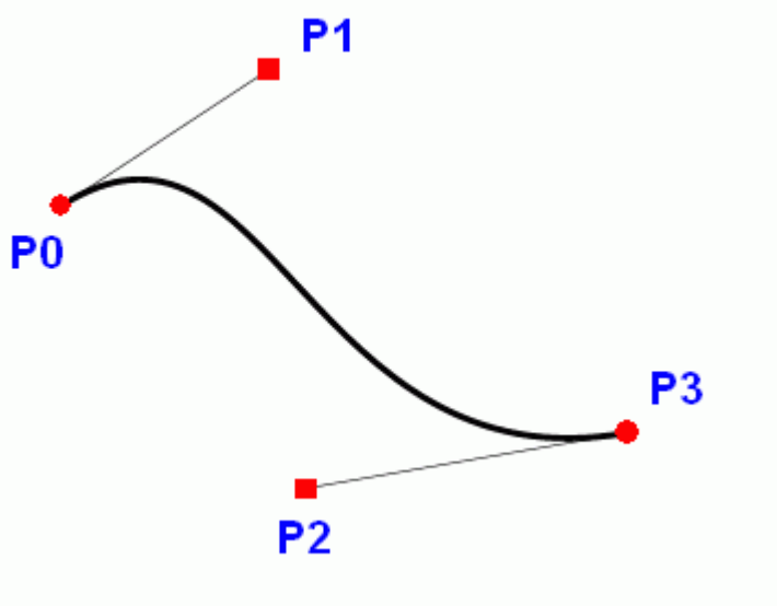
Obrázek 1.4: Kubická Bézierova křivka 1
